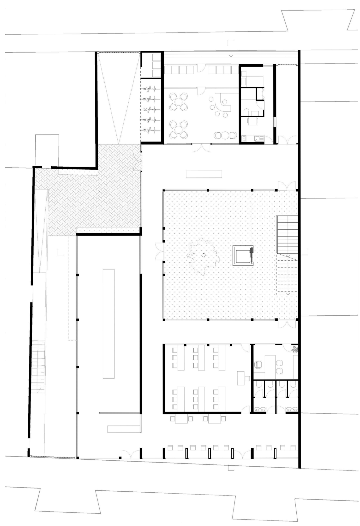
Plan RDC
