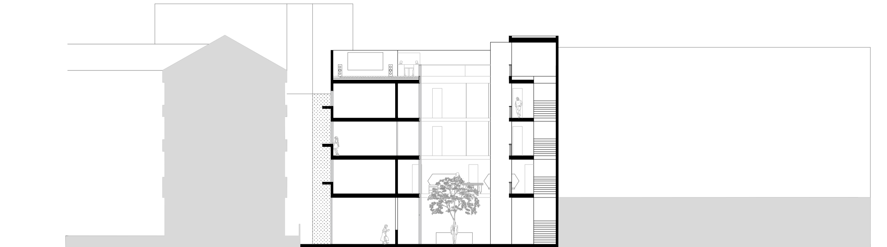
Coupe transversale
