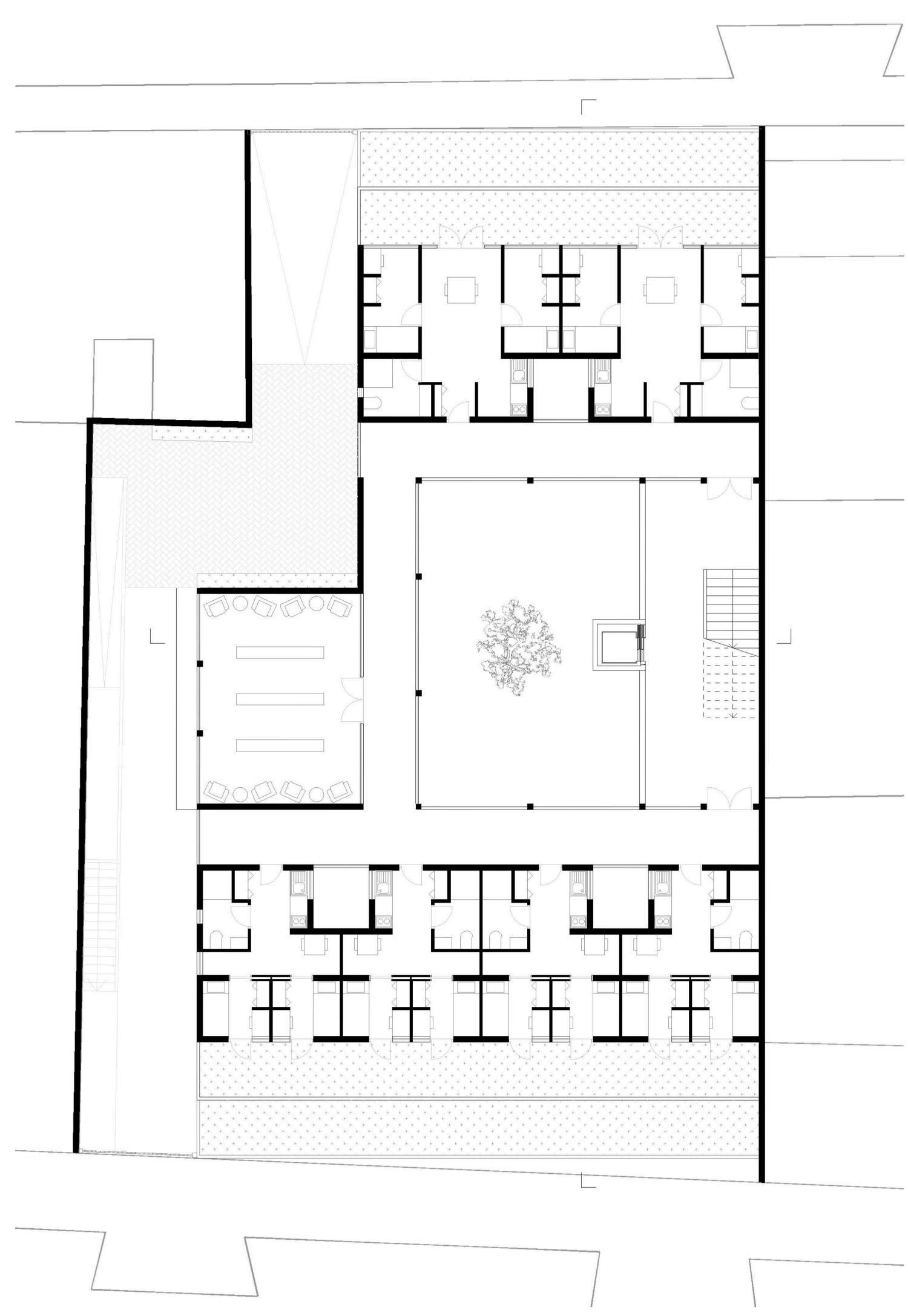
Plan R+2
