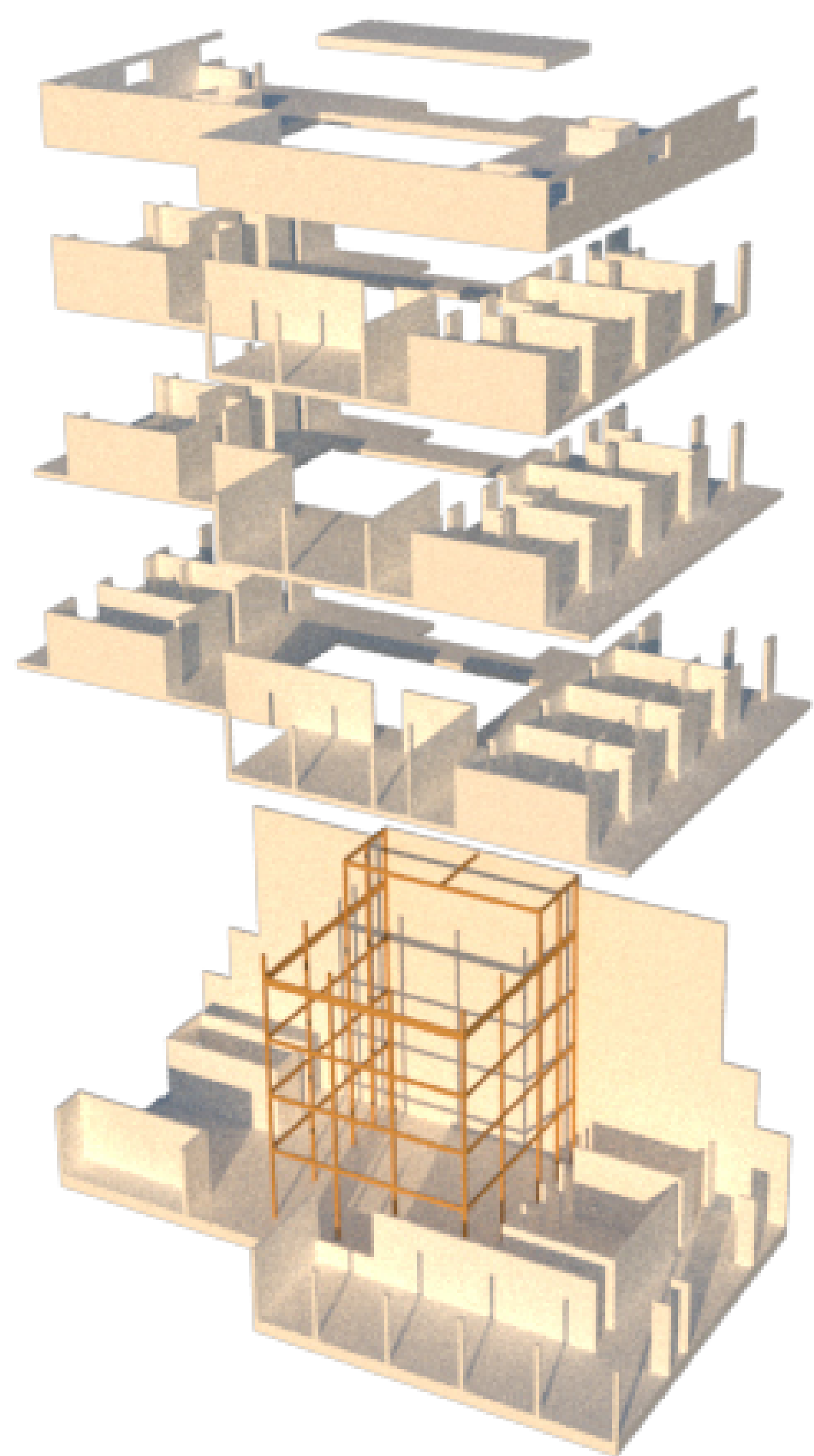
Axonométrie structure
